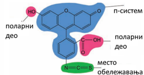
Флуоресцеин-5-изотиоцијанат
