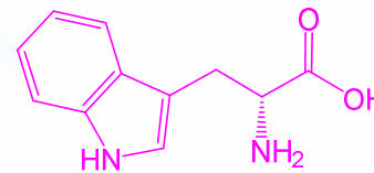
Триптофан
