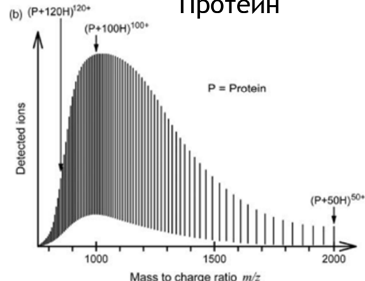
Протеин
