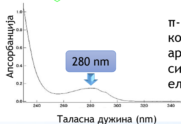
Фенилаланин
