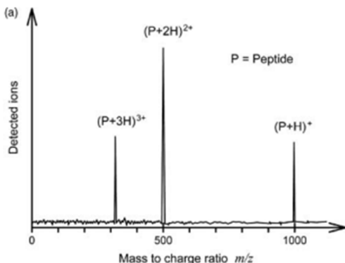
Пептид
