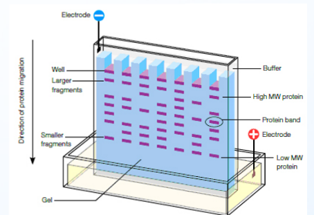
Електрофореза
