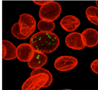
Конфокална микроскопија
