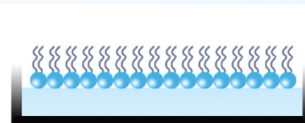
Монослој
