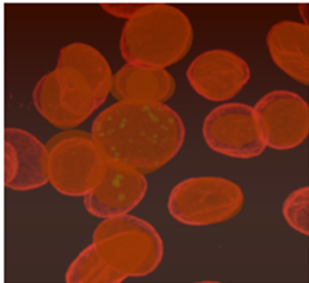
Флуоресцентна микроскопија
