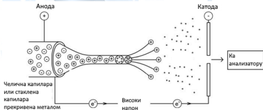
Пептид
