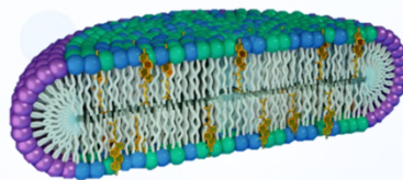
Бицеле
