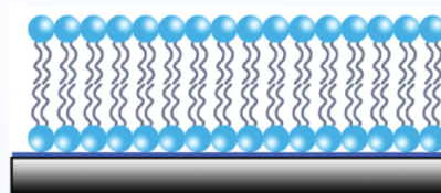
Двослој
