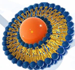
Липозоми
