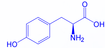
Тирозин
