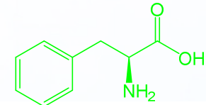
Фенилаланин
