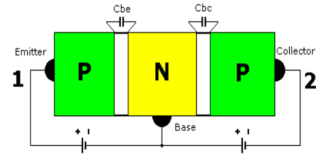
Bipolarni tranzistori
