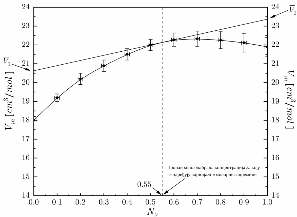
График 1. Зависност моларне запремине раствора од концентрације (молске фракције) метанола.
