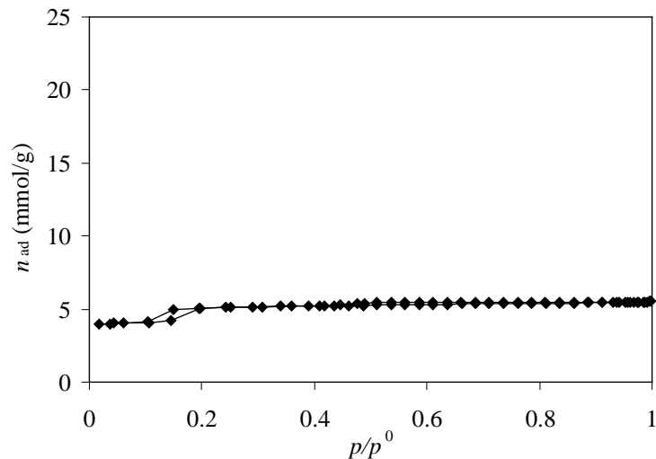
ZSM-5
