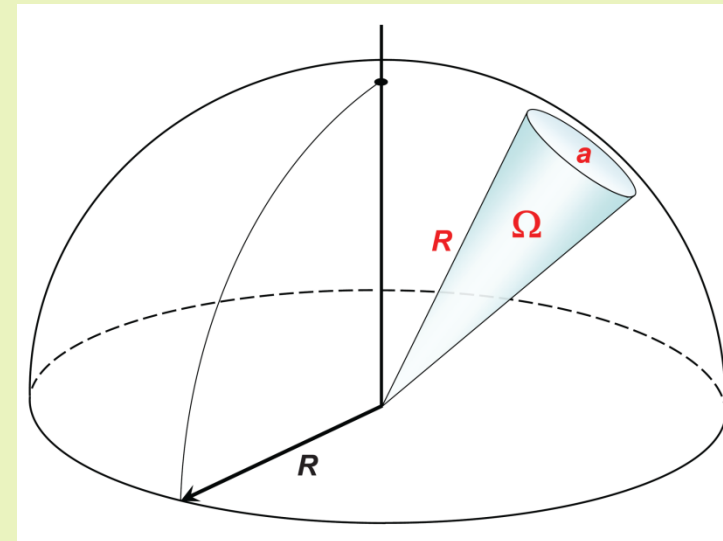
prostorni ugao
