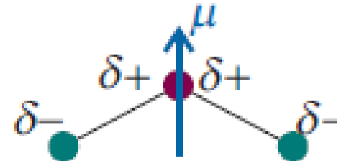
ozon, O 3
