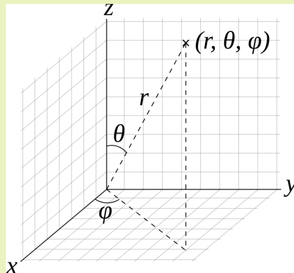
sferne koordinate
